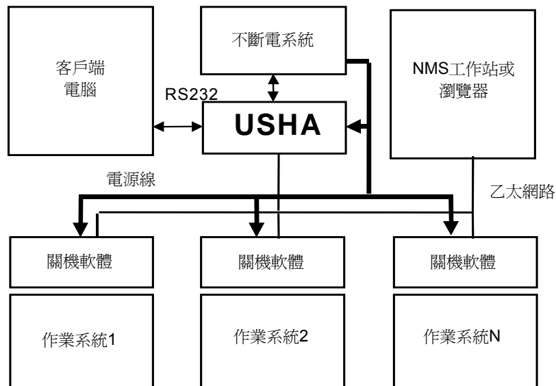
圖表1-3 USHA 系統應用圖表
