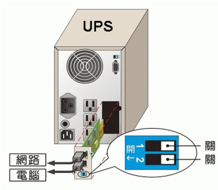
圖表2-1 USHA Card和UPS之連結
