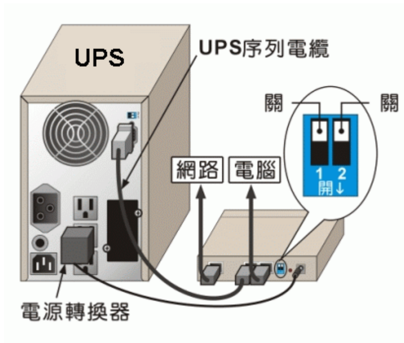
圖表2-2 USHA ProE II 和UPS的連結
